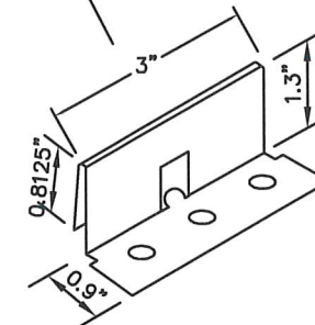
24 Ga. STEEL CLIP
