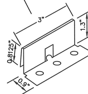
24 Ga. STEEL CLIP
