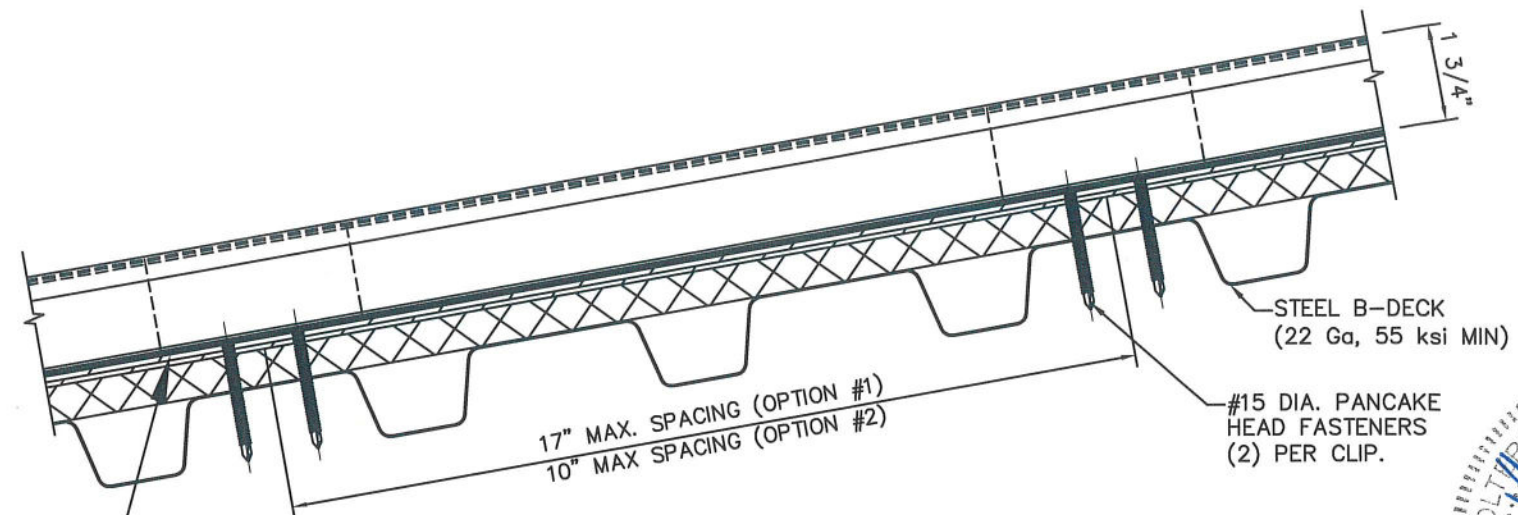
SECTION A-A
